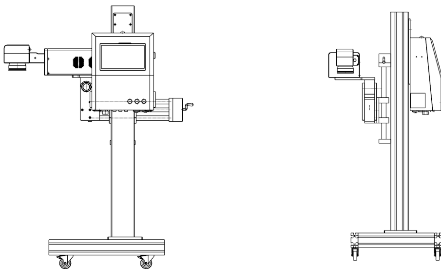
Рисунок 2-2 Система подъема главной балки для лазерной маркировочной машины
